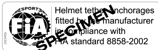
Fig 1 – Etiquette permettant d'identifier les casques équipés dès l'origine des inserts Hans®. Fig 1 – Label for identifying helmets originally equipped with Hans® inserts.
